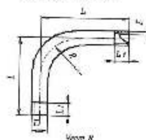
ОТВОД 90° РЕЗЬБОВЫЙ
